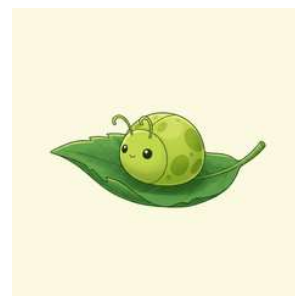
bug
